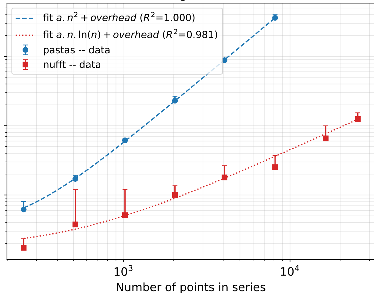
rectangle kernel
